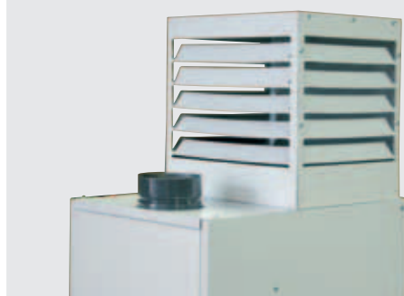
Plénum pour soufflage direct à 3 faces (fabrication sur demande)
